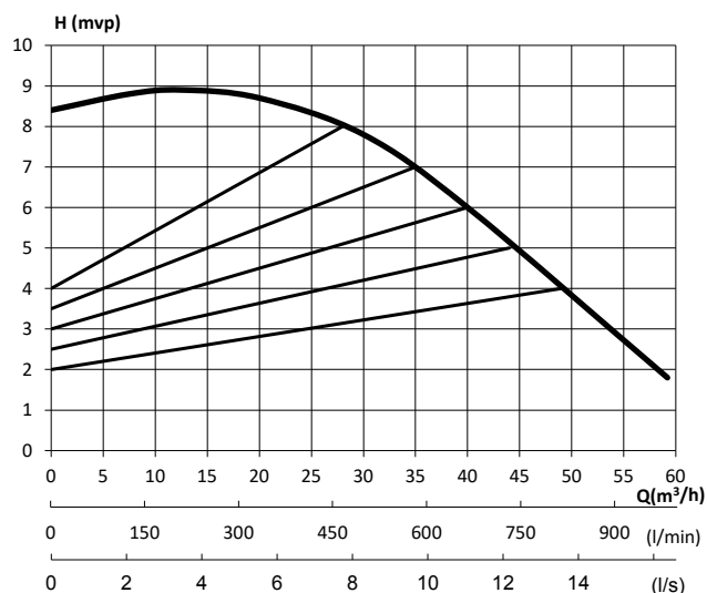
Kapacitetsdiagram 100-18/73
