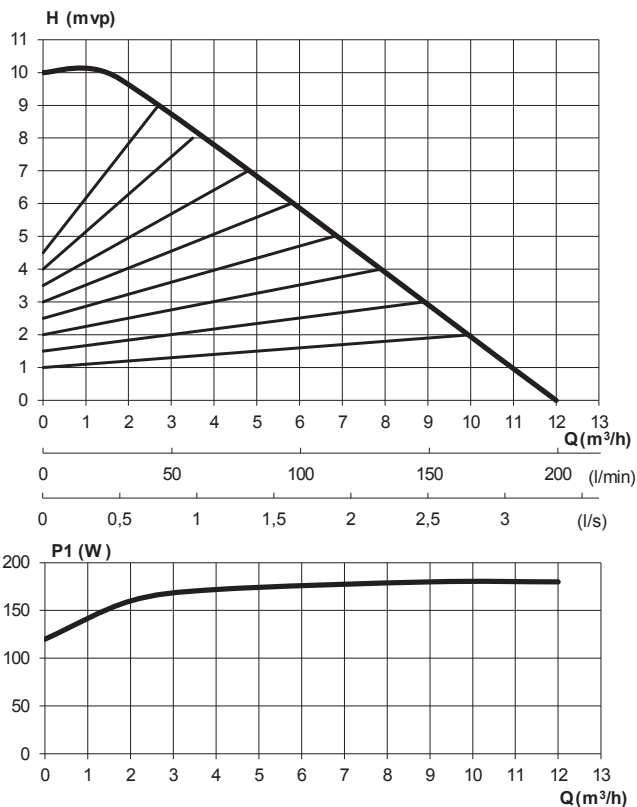
Kapacitetsdiagram 25-50 -10/12
