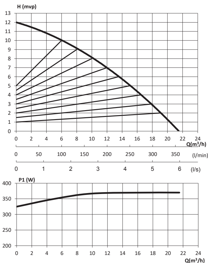
Kapacitetsdiagram 32F-12/21
