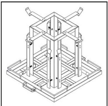
WD209.7364 Kassett för 500x500 diskorg
