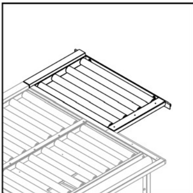
WD209.7375 Anslutningsbana, speciallängd, l = 180 - 840 mm (beställs i samband med diskmaskinsbeställning)
