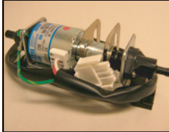
Diskm. pump GRI 14825 m. kontakt 716,0501
