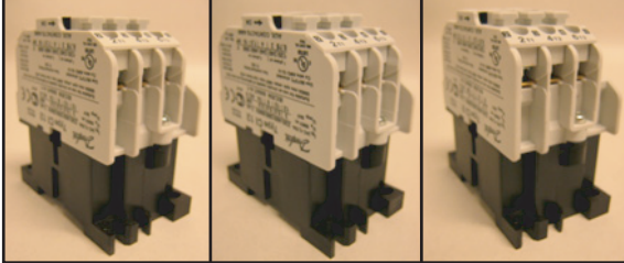
Kontaktor CI12 220-240V/50 20A 63723133
