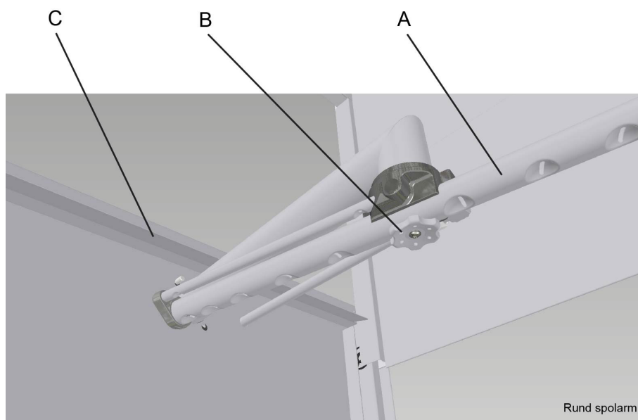
A=Övre diskarm B=Låsmutter C=Stänklis
