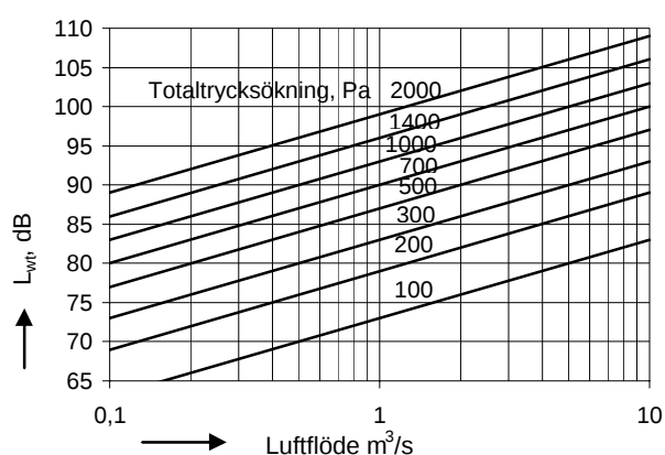
Total ljudeffektnivå, L_{wt}
