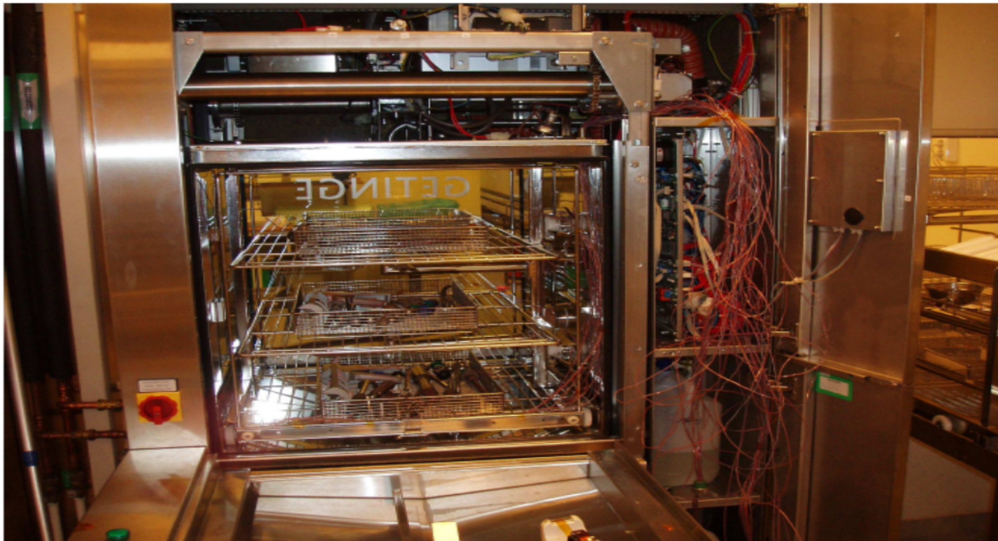
Givarna placerade i maskin
