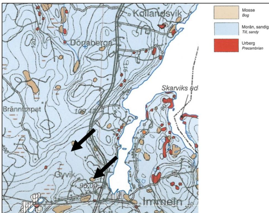
Utsnitt ur SGU:s jordartskarta där läget för vattentäkterna är ungefärligt markerade med svarta pilar.
