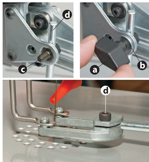
Saw guard assembly (d) assembled
