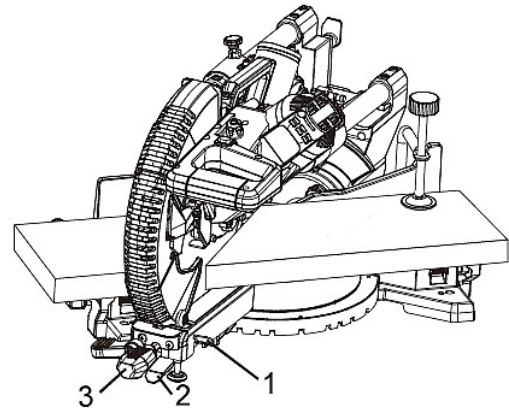
Fig. 38: Mitre cut
