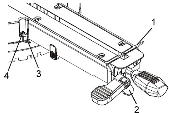
Fig. 21: Mitre scale
