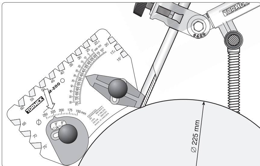
Inställning av en skålskölp med 45° eggvinkel i SVD-186 jiggen. Slipskivans diameter är 225 mm.
