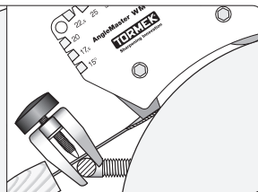
Inställning av en ny eggvinkel kan antingen göras med ögonmått eller till en viss bestämd vinkel med vinkelmätaren WM-200 (sidan 142).
