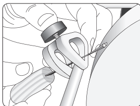
Slipa bara där ljuslinjen är som tjockast medan du låter verktyget rulla på universalstödet. Kontrollera ofta var slipningen sker. Slipa tills att du får en jämn och tunn ljuslinje.
